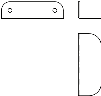
Top Door Strike Plate
